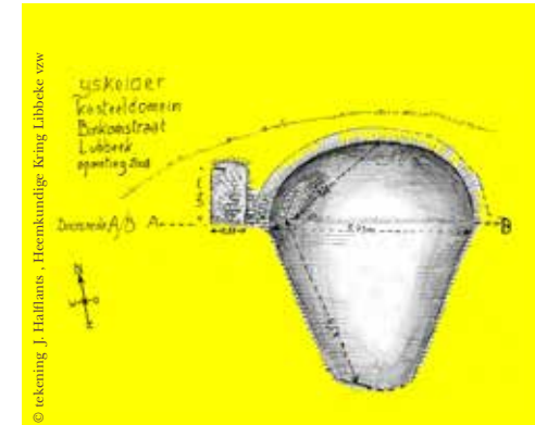
Plan en doorsnede van de ijskelder op het kasteeldomein 't Serclaes
